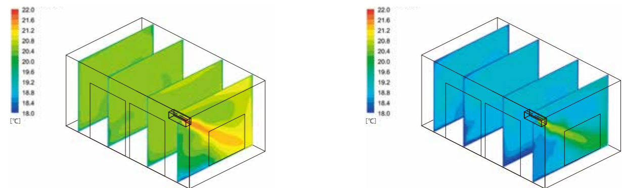
超高断熱真空ガラス 「スーパースペーシア」(Low-E4ミリ+真空層0.2ミリ+フロート板ガラス4ミリ)
